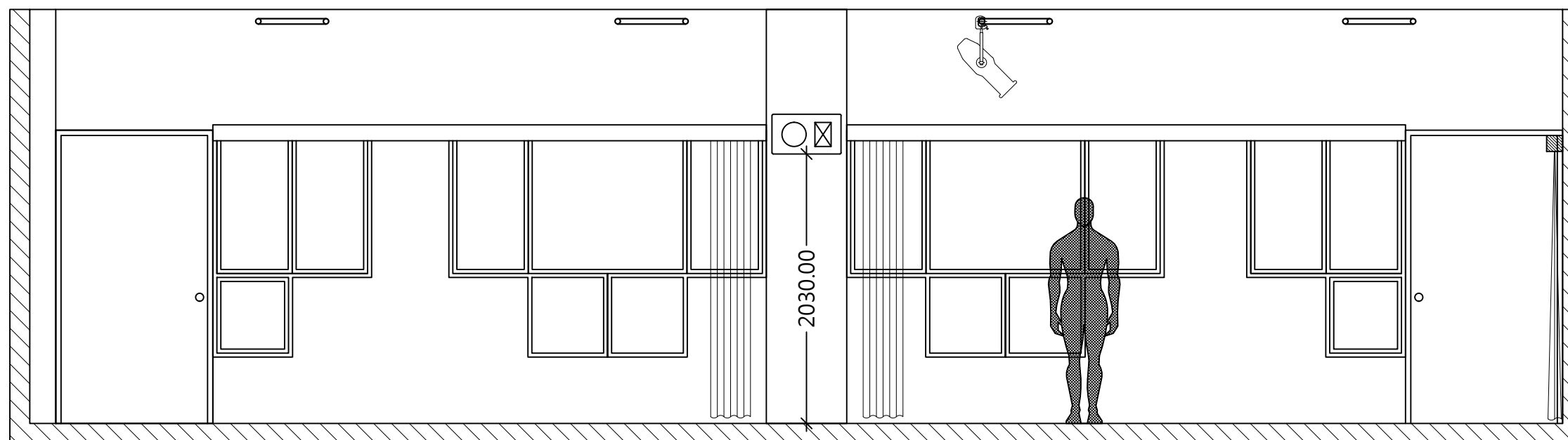
2 右視圖 S-1.0
