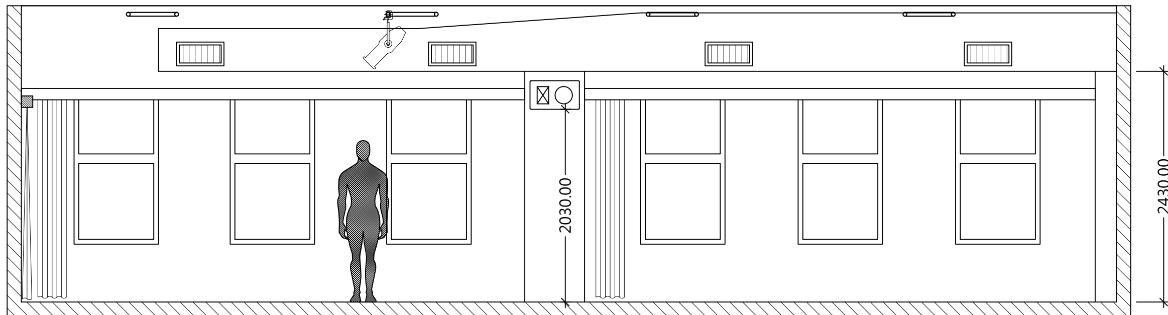
1 左視圖 S-1.0
